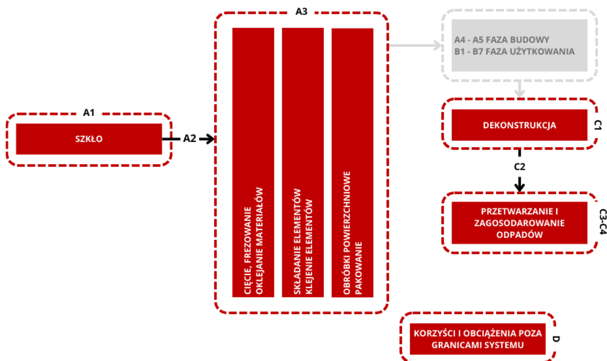
Rysunek 5.1: Granice systemu dla charakterystyki środowiskowej drzwi szklanych
